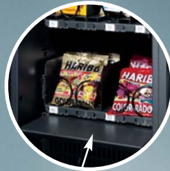
Motorisierte Diebstahlsicherung
